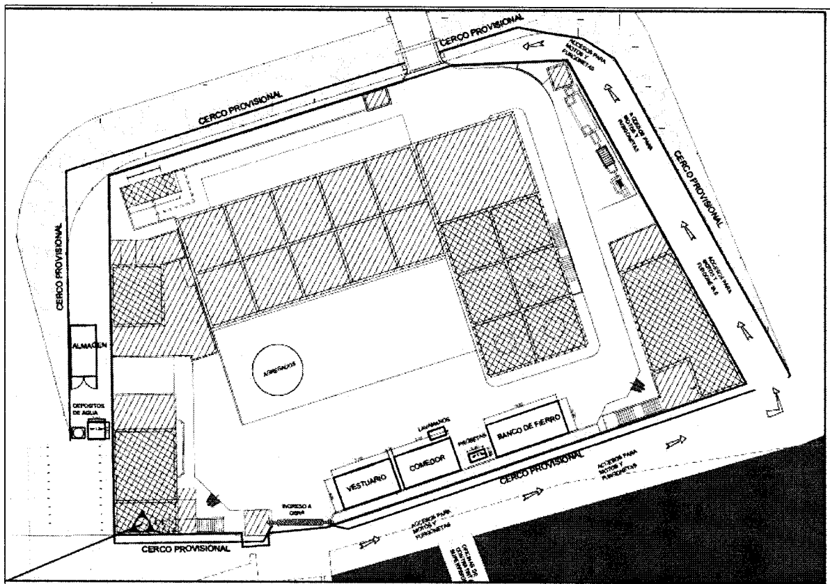
Imagen 1.- layout de obra, se muestra la ubicación, medidas de las obras provisionales
